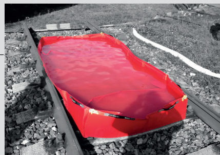
Vanu je možné umístit pod vlak nebo jiné drážní vozidlo dvěma způsoby: napříč přes koleje nebo podélně do vnitřního prostoru mezi kolejemi. Oba způsoby použití byly podrobeny náročným testům.
