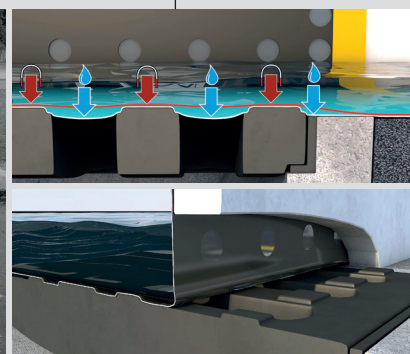
Detail funkce hydrostatického tlaku
